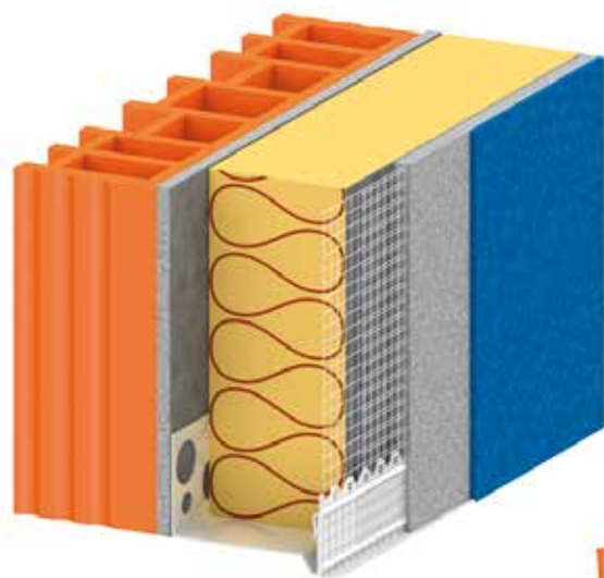
Detail okapnice s tkaninou pro soklový profil
