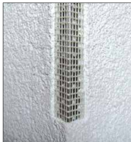
Detail umístění kombi lišty - řez
