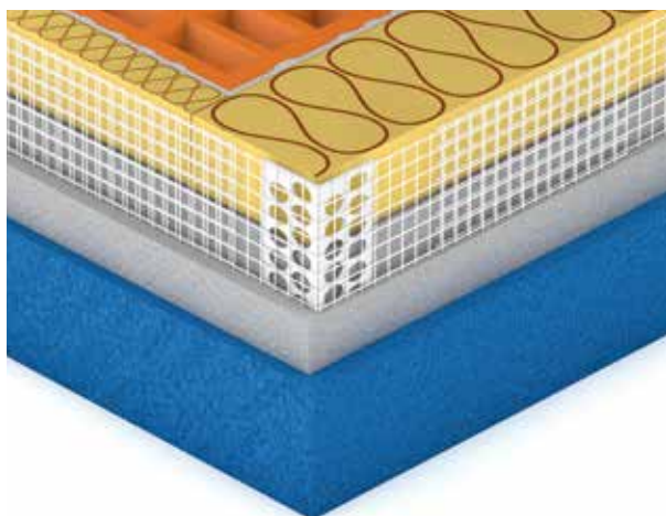
Aplikace rohové lišty s tkaninou
