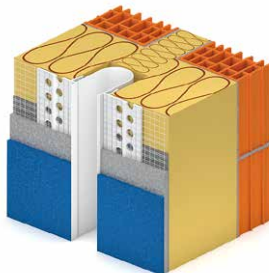
Dilatační profil stěnový (E)
