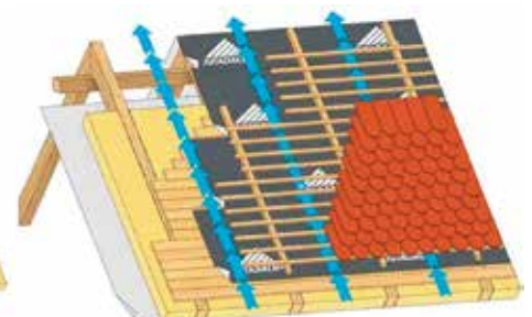
Skladba tříplášťové střechy s bedněním
