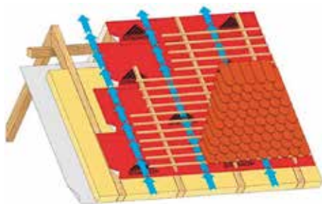
Skladba dvouplášťové střechy bez bednění
